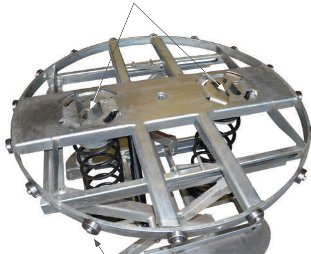
Ouverture pour changer les ressorts facilement
